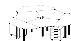
3 fős munkahely / 3-Person Arbeitsplatz / 3 person work station Befoglaló méret / gesamte Größe / Space required: 2800x2800x720
