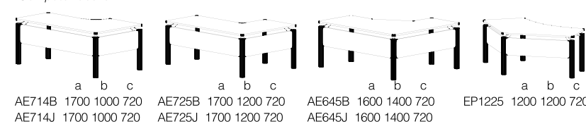
Számítógépes asztalok Computertische Computer desks
