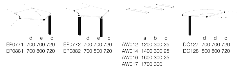
Tárgyalóasztalok Besprechungstische Conference tables
