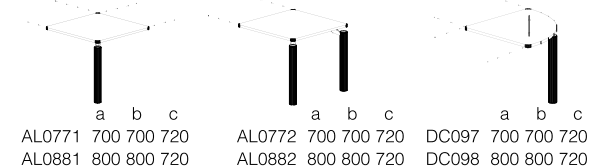
Sarokasztalok Ecktische Corner tables
