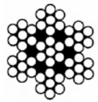
Edelstahl-Drahtseil 7x7 DIN 3060
